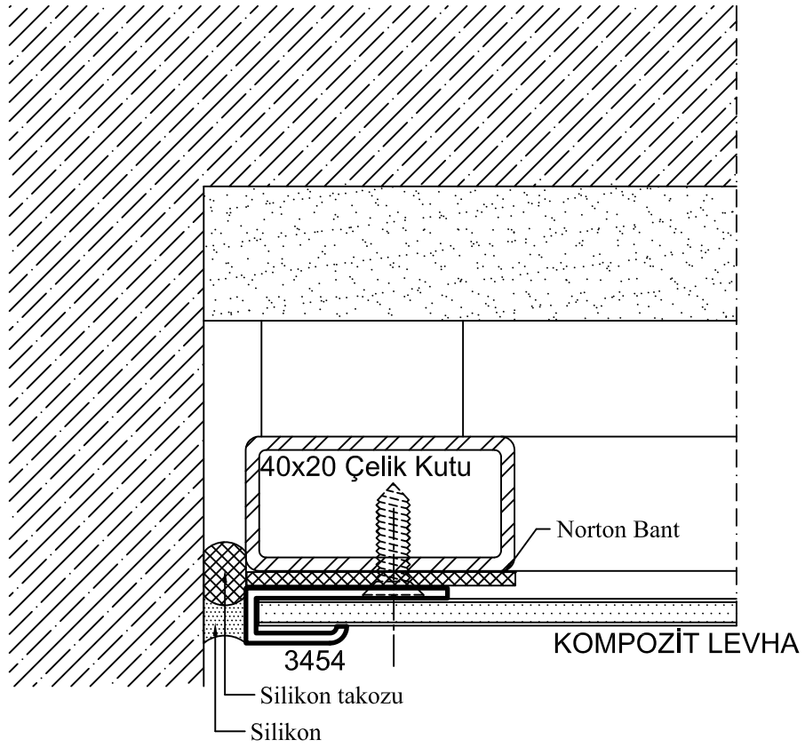
7 DETAYI
